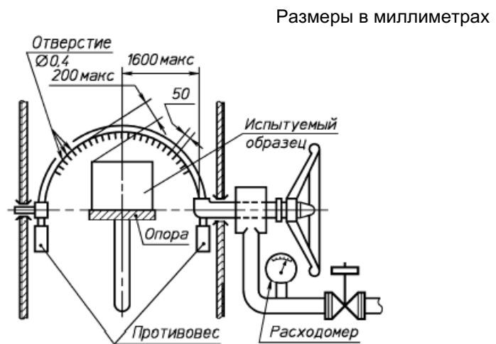
Рисунок 3 - Устройство для проверки защиты от вертикально падающих капель воды (емкость для получения капель)
