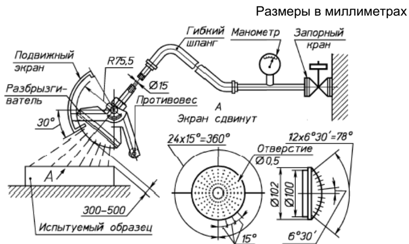
Рисунок 4 - Устройство для проверки защиты от дождя и обрызгивания водой; вторые характеристические цифры 3 и 4 (качающаяся труба)
